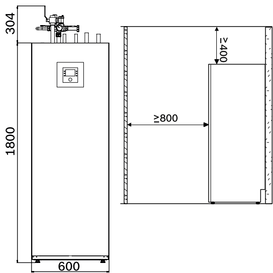
Unidad interior AWM (acumulación)
