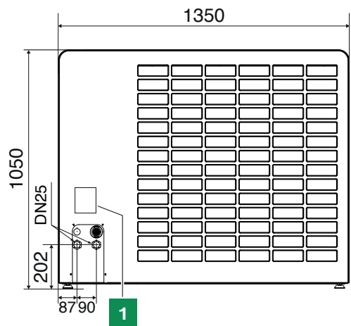
Dimensiones y conexiones de la bomba de calor, parte trasera
