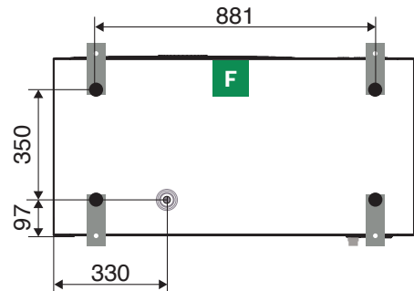
Distancias al conector de vaciado, vista inferior
