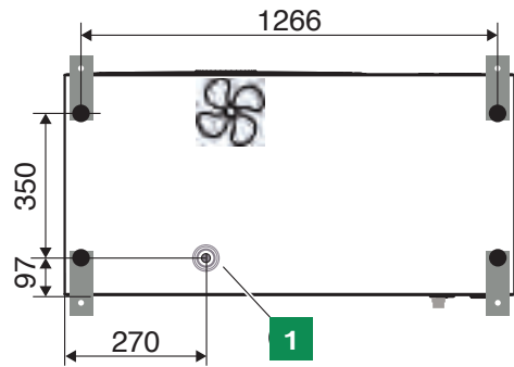
Distancias al conector de vaciado, vista inferior
